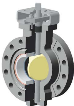
Рис. 29. затвор дисковый РУСТ® серии 800
