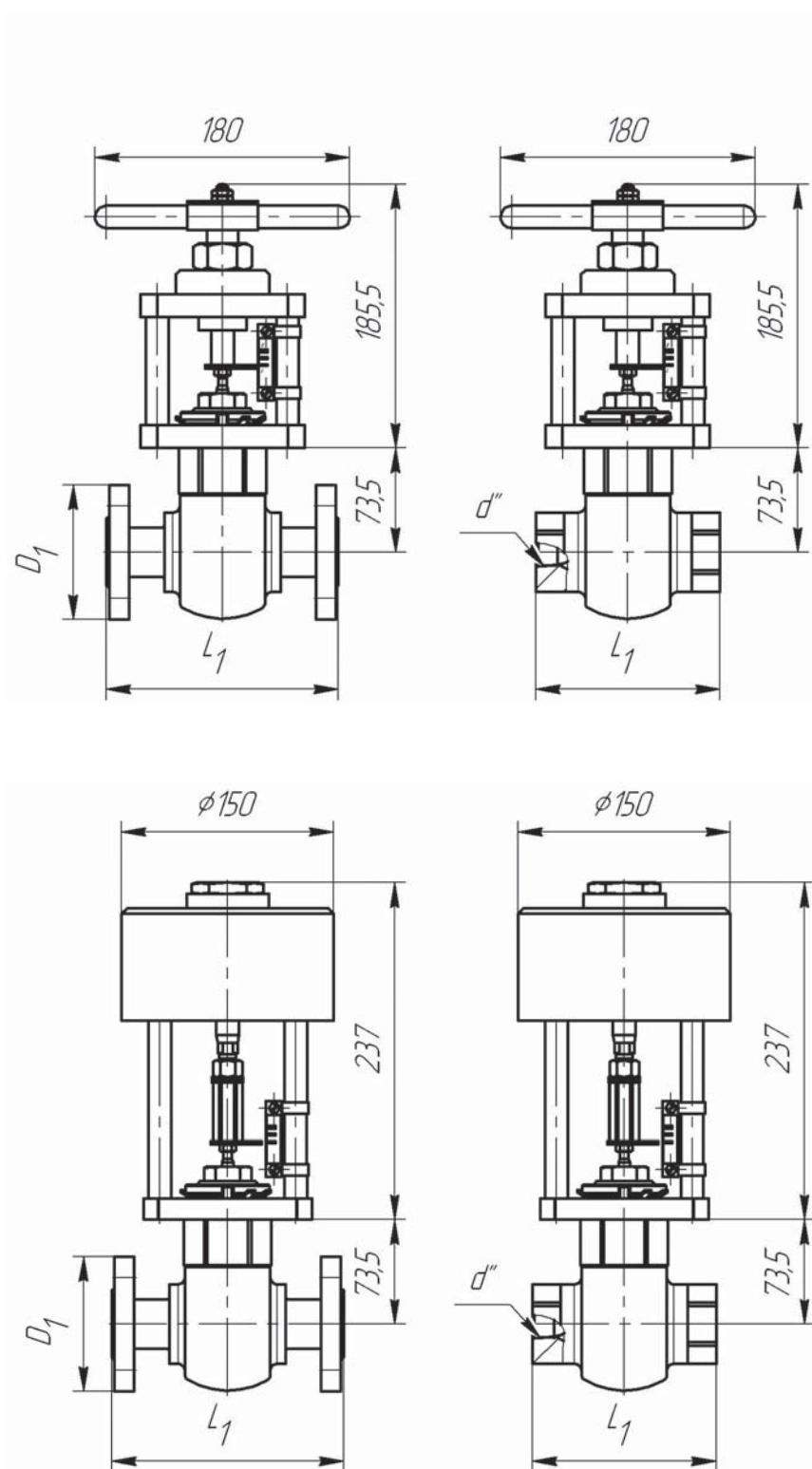
Рис. 20. Габаритные размеры клапанов микрорасхода РУСТ серии 411
