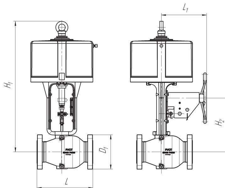
Рис. 40. Габаритные и присоединительные размеры клапанов осевых РУСТ® серии 900 с поршневыми приводами
