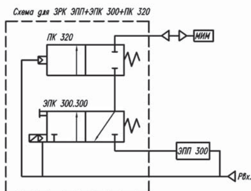
Рис. 61. Габариты и пневмосхема ПК 320
