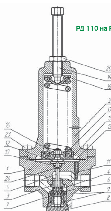
Рис.46. Конструкция регулятора давления РД 110
