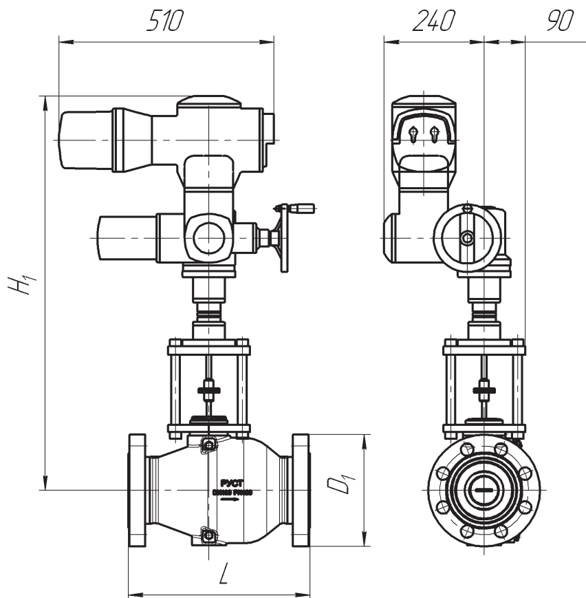
Рис. 41. Габаритные и присоединительные размеры клапанов осевых РУСТ® серии 900 с электроприводом АУМА
