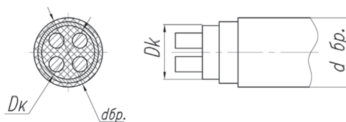
Рис.68 Dk – диаметр уплотняемого кабеля; dbp – диаметр брони кабеля (для ВКВ 070)
