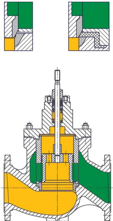
Рис. 4. Исполнения основного уплотнения клапанов РУСТ® серий 300, 400, 500
